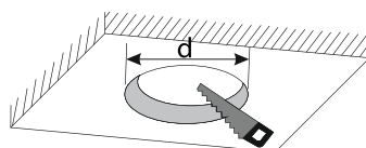
Рис.2. Врезное отверстие
