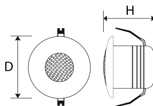
Рис.1. Габаритные размеры
